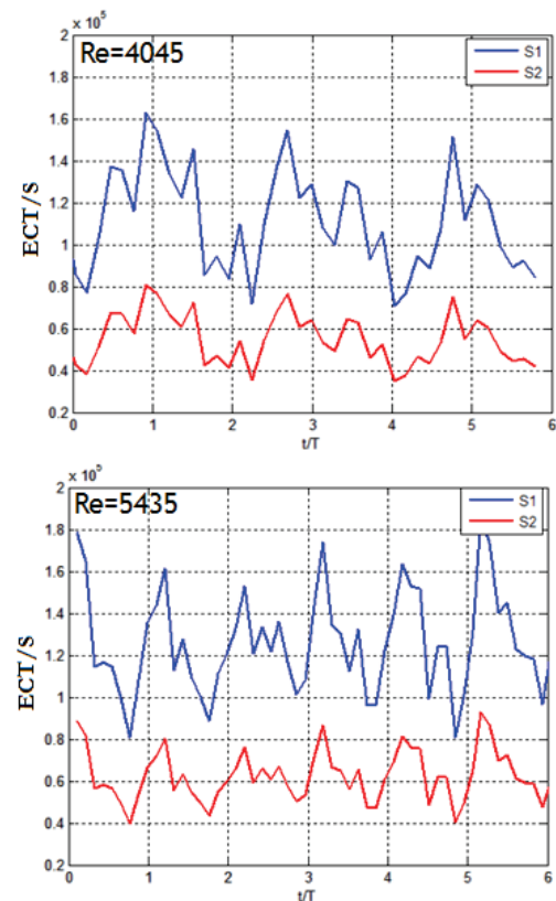
Figure 4. Amplitudes normalisées du signal acoustique et de l'énergie cinétique turbulente bidimensionnelle par unité de surface et par cycle acoustique T . L/H=4
